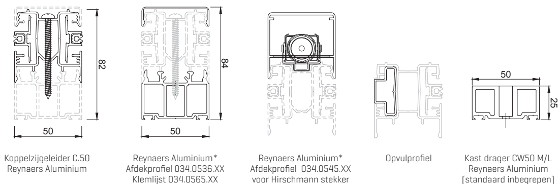
Zijgeleiders
